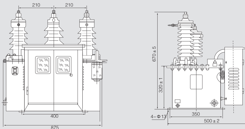
图 1：6kV、10kV、11kV 三相四线油浸式高压电力计量箱（三相三元件）
