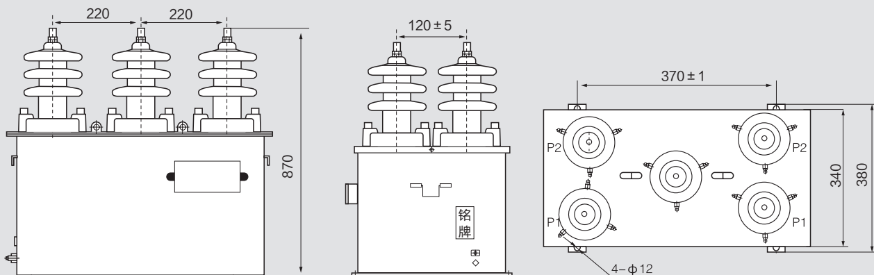
JLSZV8-6、10 瓷瓶伞群式
